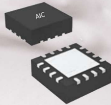
QFN-16(3x3)
